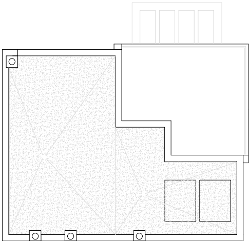
PLANTA CUBIERTA.
