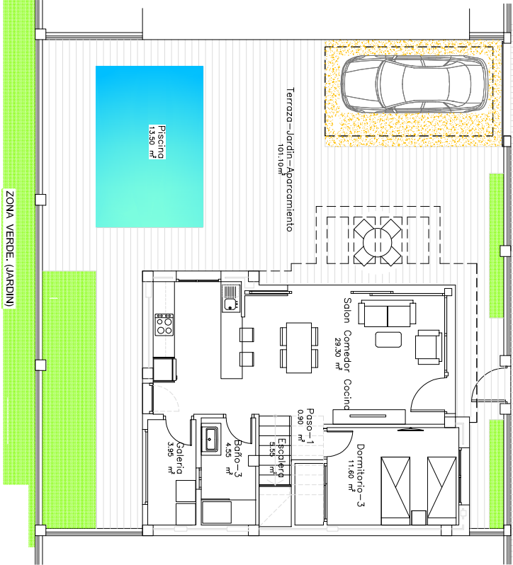
PLANTA BAJA.
